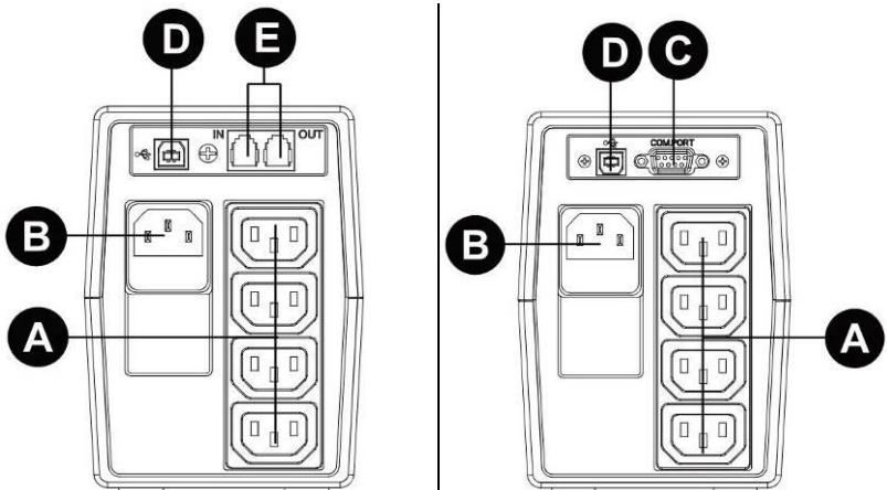
Darstellung der Geräte-Rückseiten: 400, 600, 800 VA
